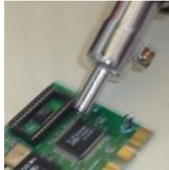
Resim 3.4: Isı Havyası ile lehim sökölmesi
