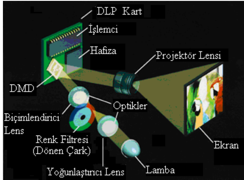
Şekil 1.16: Projeksiyon TV yapısı
