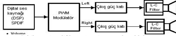
Şekil 1.8: Amplifikatör/receiver güç katı blok şeması
