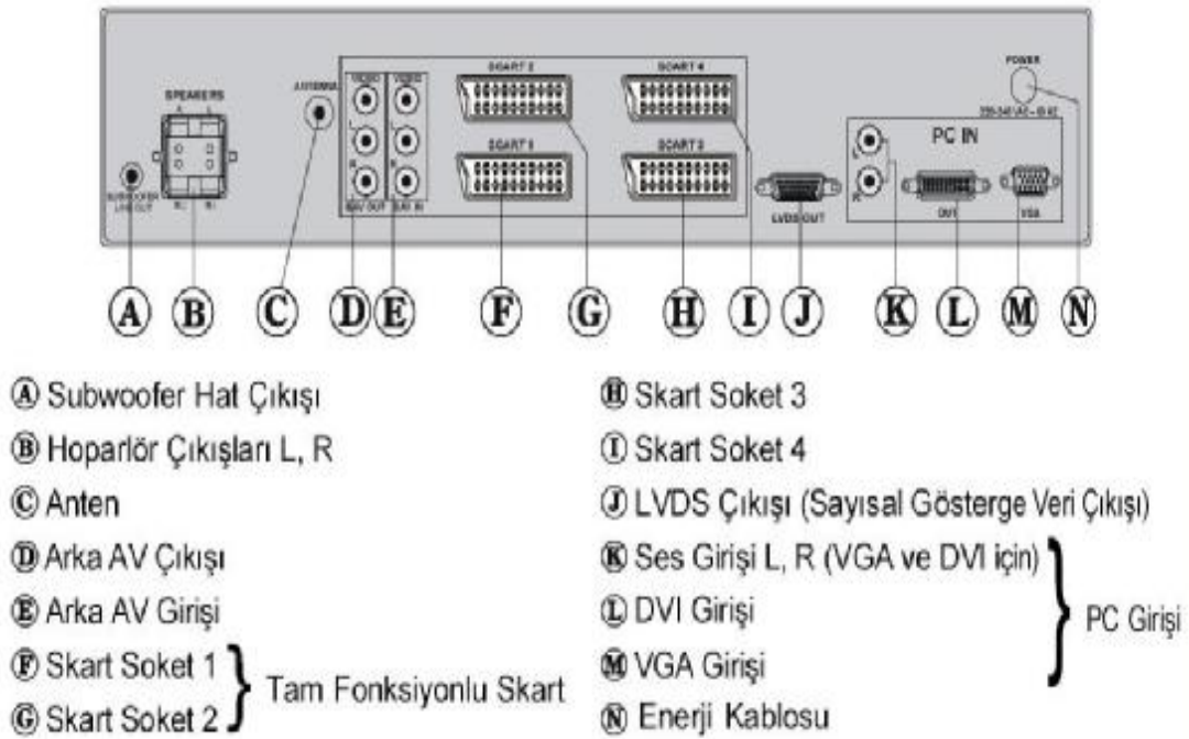
Şekil 1.18: Plazma TV giriş-çıkış bağlantıları
