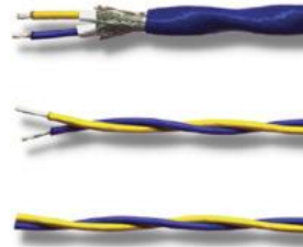
Şekil 1.12: Twisted pair dijital ses kablosu
