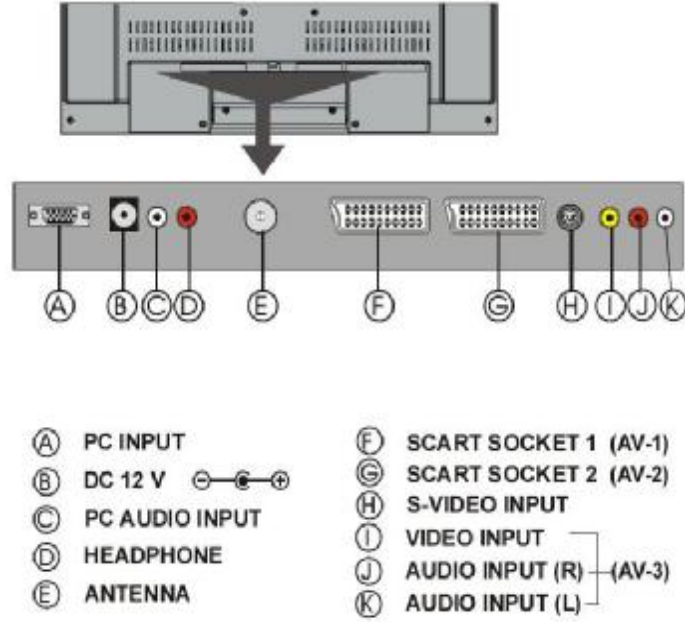
Şekil 1.21: LCD TV giriş-çıkış bağlantıları
