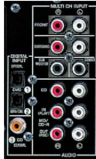
Resim1.2: Amplifikatör/receiver audio (ses) girişleri
