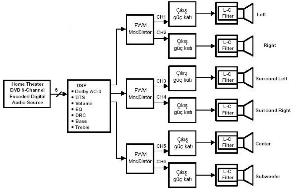
Şekil 1.10: Amplifikatör/receiver 6 kanallı ses katı blok şeması
