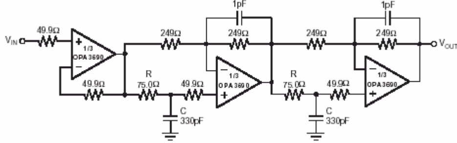
Şekil 1.4: Amplifikatör/receiver preamplifikatör devresi
