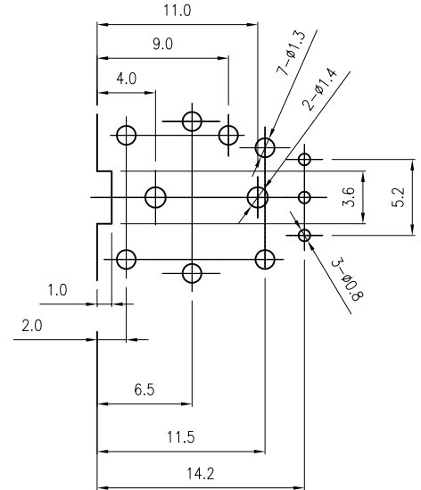
P.C.B LAYOUT
